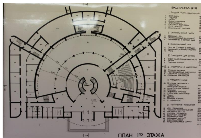
Рисунок 7.5 – План 1го этажа.
