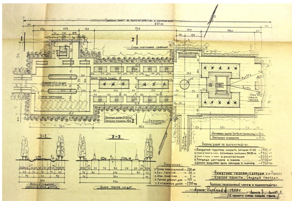
Рисунок 2.2 – Генеральный план, разбивочный чертёж и благоустройство.
