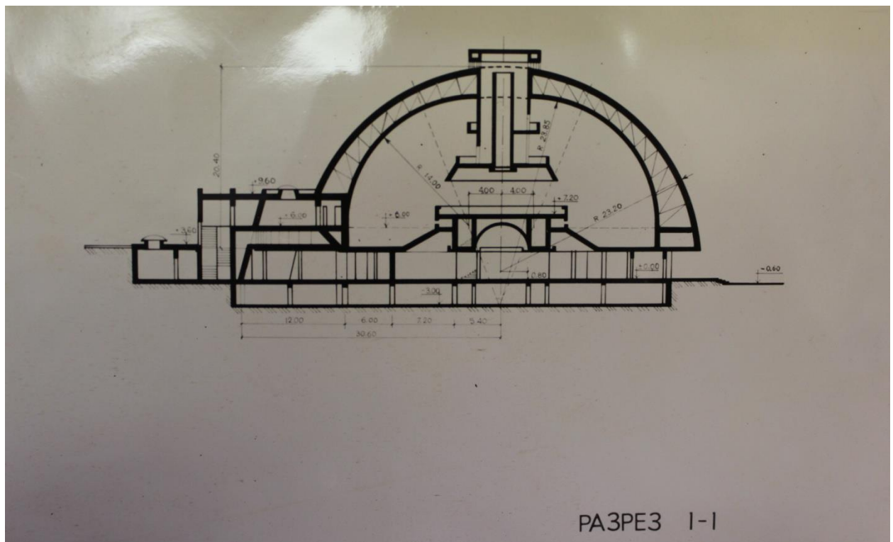
Рисунок 7.7 – Разрез 1-1.
