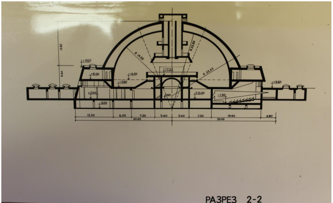
Рисунок 7.8 – Разрез 2-2.
