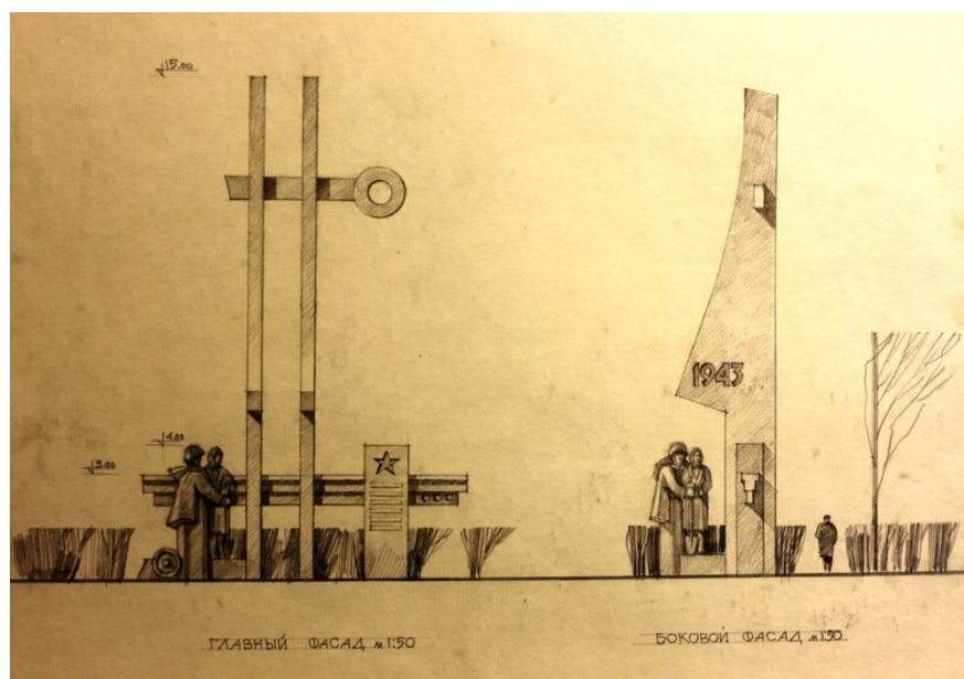
Рисунок 3.6 – Главный и боковой фасад варианта 3.
