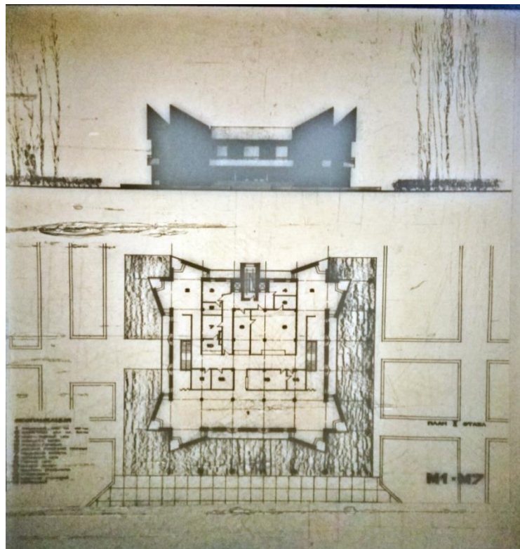
Рисунок 5.4 – Проект вспомогательного здания на территории мемориального комплекса.
