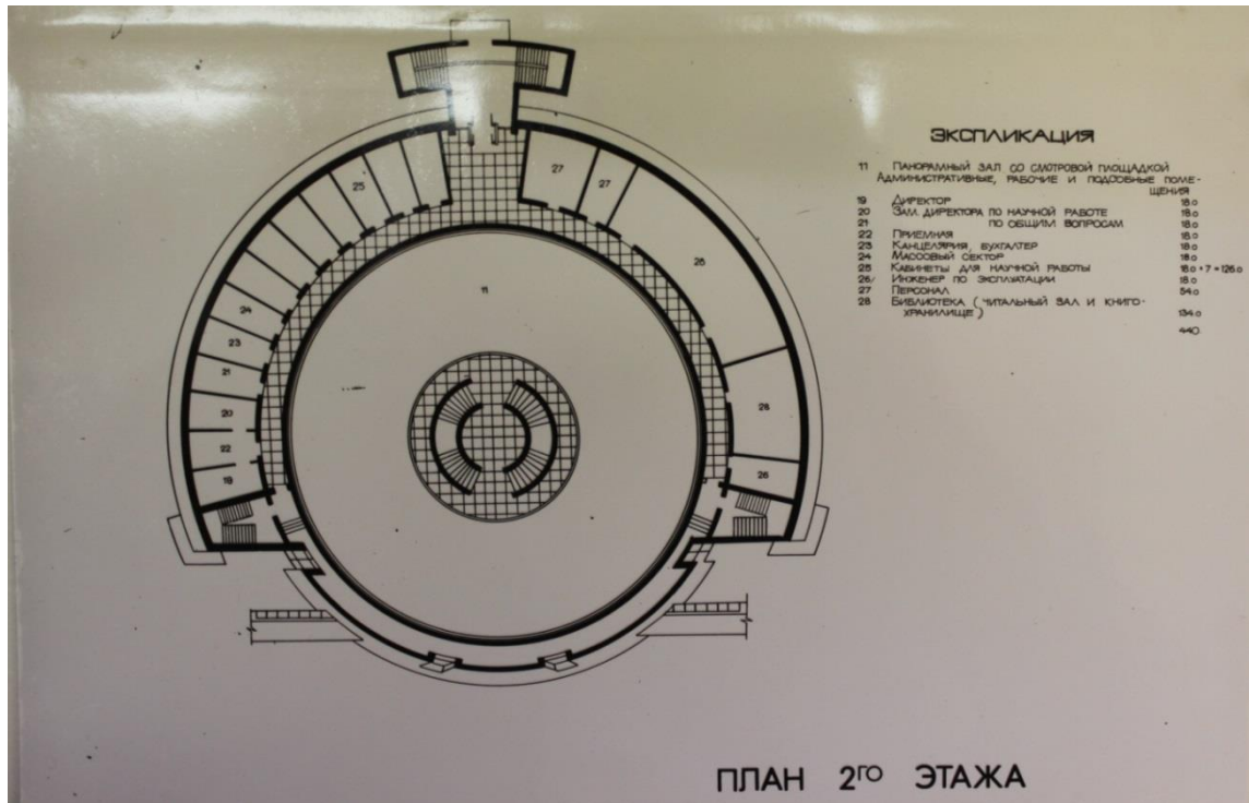
Рисунок 7.6 – План 2го этажа.
