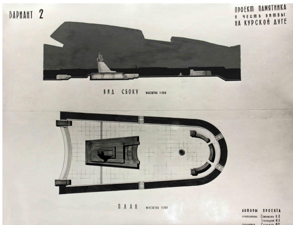
Рисунок 4.4 – Вариант 2
