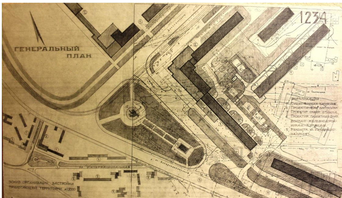
Рисунок 3.7 – Генеральный план проекта памятника Воинам-железнодорожникам по ул. Интернациональной.
